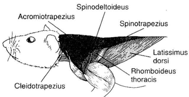
Hamster
