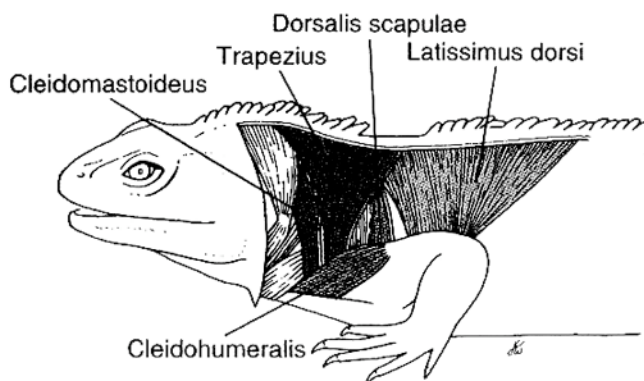
Sphenodon
