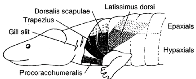
Necturus
